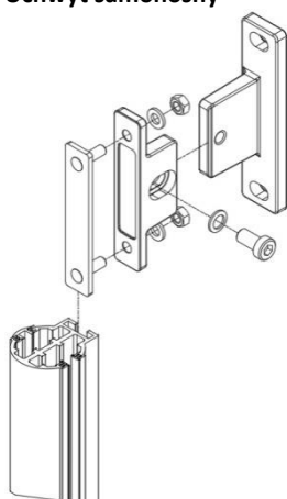
Prowadnica OVAL (okrągła)
