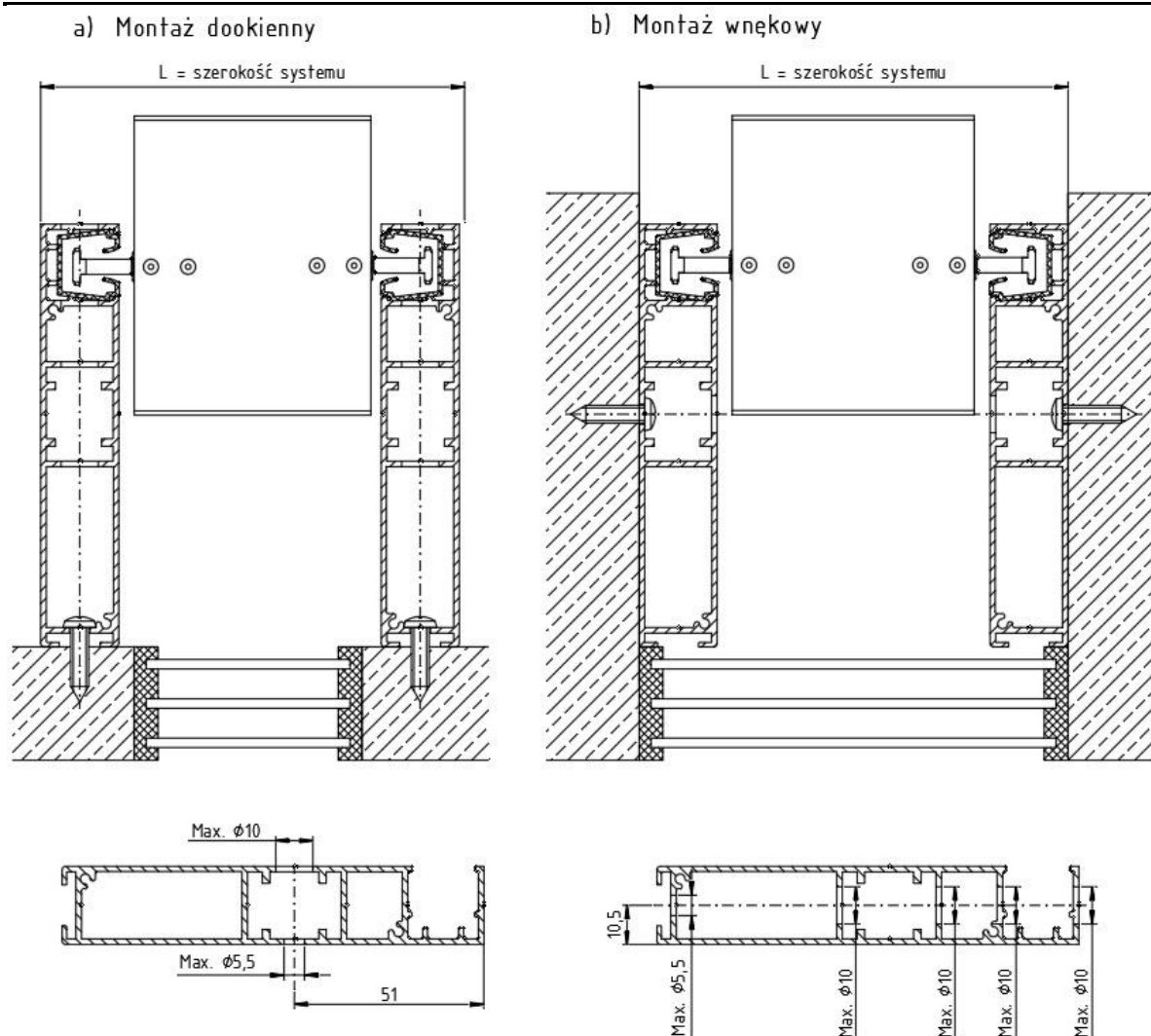
Rys. 12. Sposoby montażu prowadnicy: a) – Montaż dokienny b) - Montaż wewnętrzny
