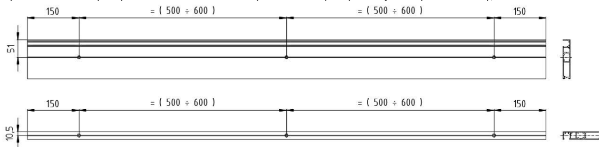
Rys. 13. Schemat wykonywania otworów montażowych w kasecie podtynkowej. * - Wymiar zmienny, standardowo 30 mm.
